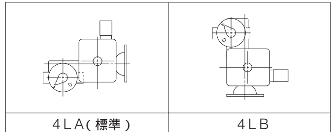
三相電動機(4L)取付け方向
