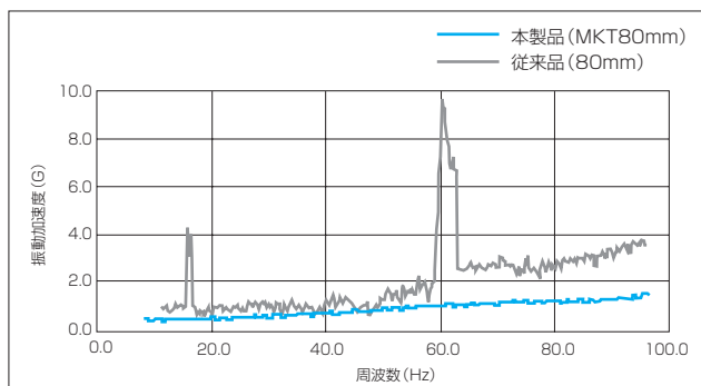
上図のように、あらゆる周波数域で振動ピークが無く、振動による損傷を防ぎます。
