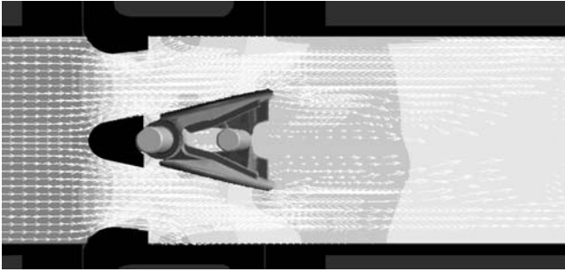
注)色は圧力分布を示します。赤色は高圧部、青色は低圧部です。矢印の大きさは流速の大きさを示します。 高圧 ←————→ 低圧
